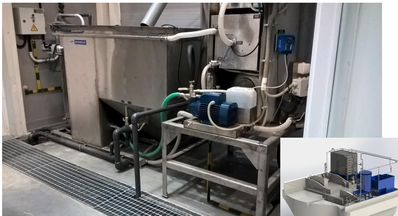
Камера гидроиспытаний.
